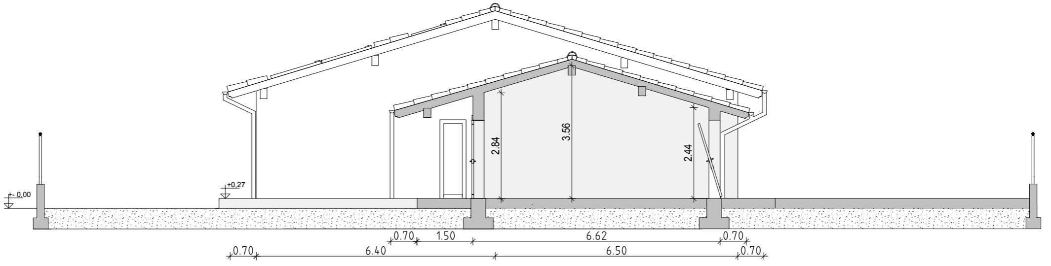
Sezione C-C
