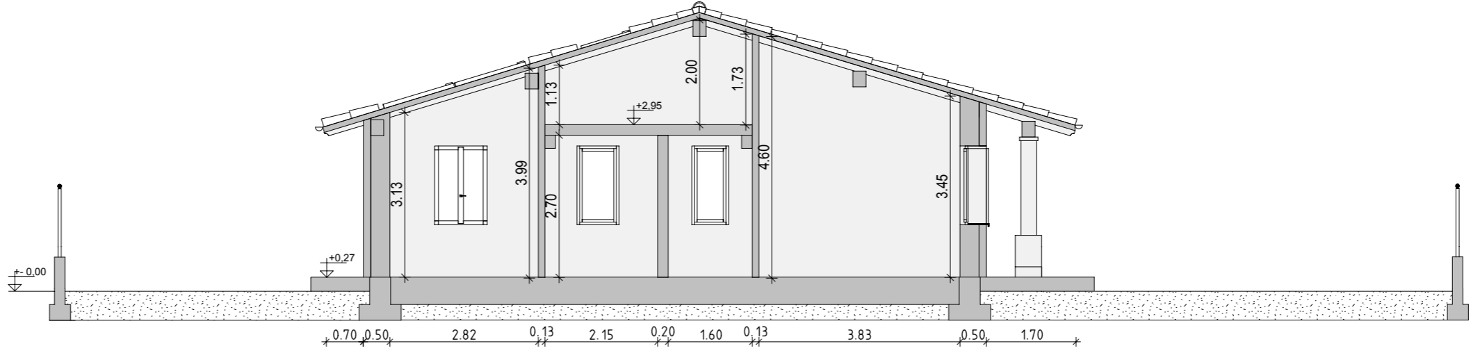
Sezione A-A
